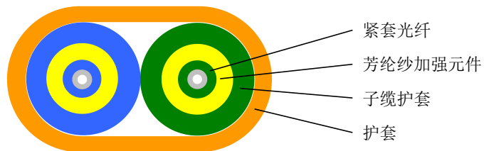
双芯扁形室内光缆 II 型
